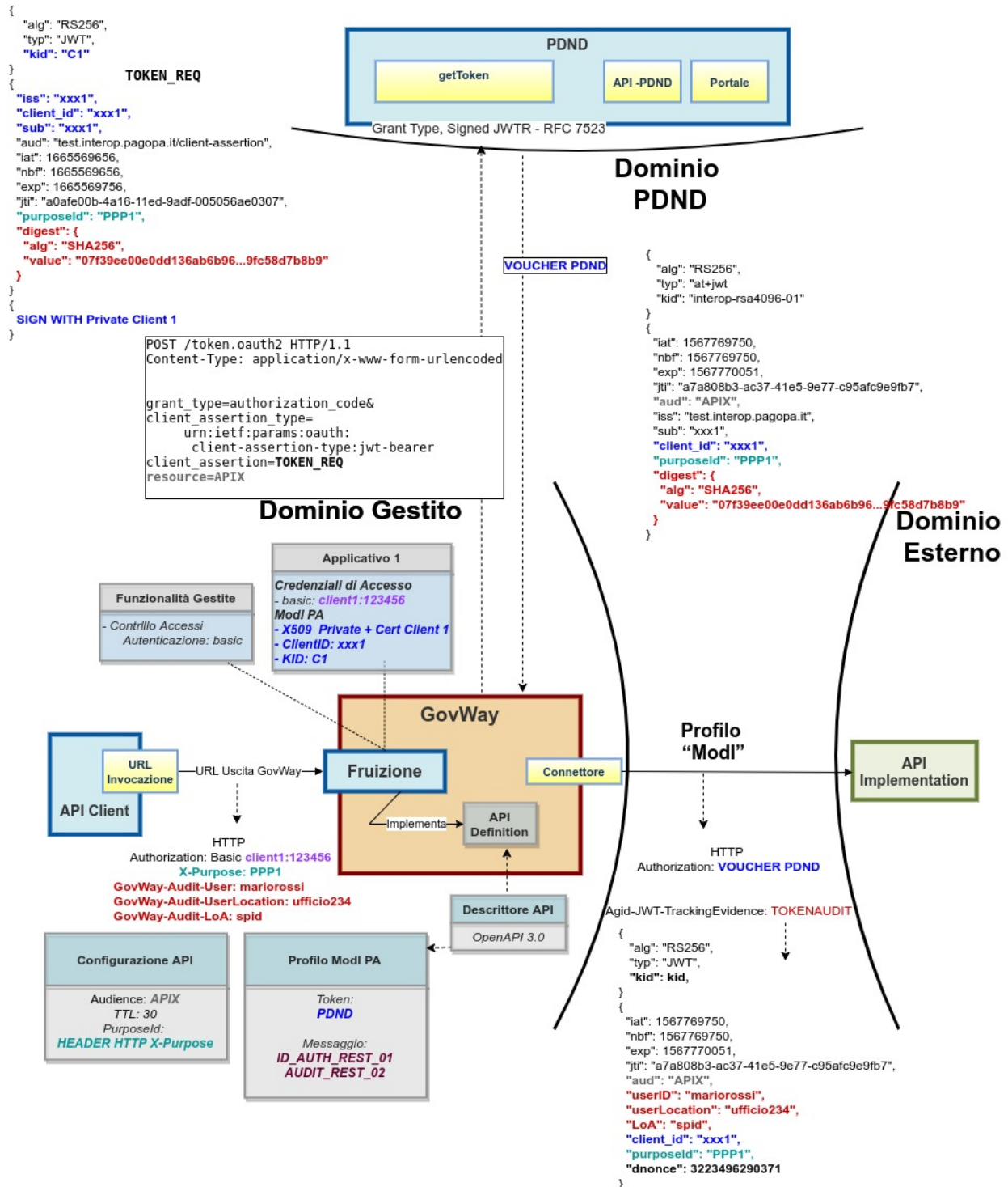
Fig. 3.99: Profilo di Interoperabilità "ModI", pattern "AUDIT_REST_02": trust tramite PDND
