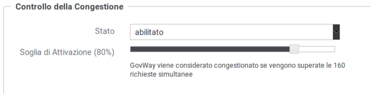
Fig. 8.34: Configurazione della soglia di congestionamento
