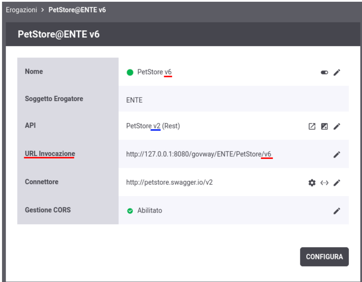
Fig. 10.7: Nuova versione dell'erogazione differente dalla versione dell'API
