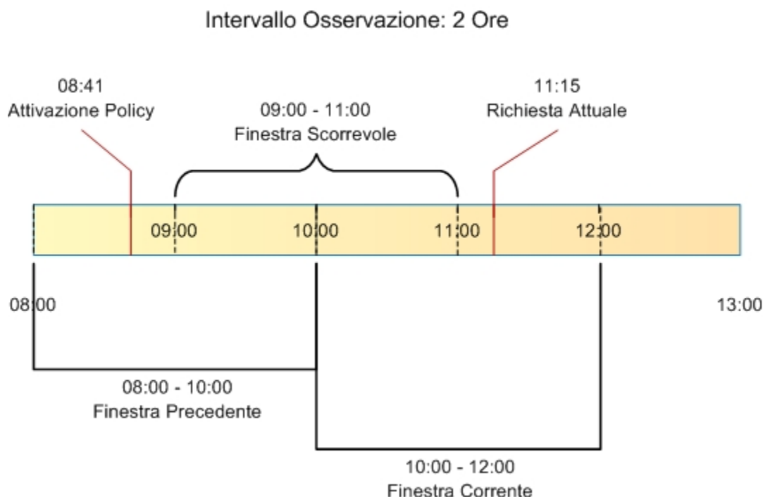
Fig. 8.37: Finestre di osservazione su un campionamento di 2 ore
