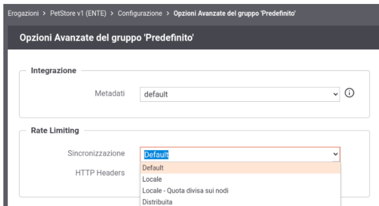
Fig. 2.103: Sincronizzazione del Rate Limiting in un cluster di nodi
