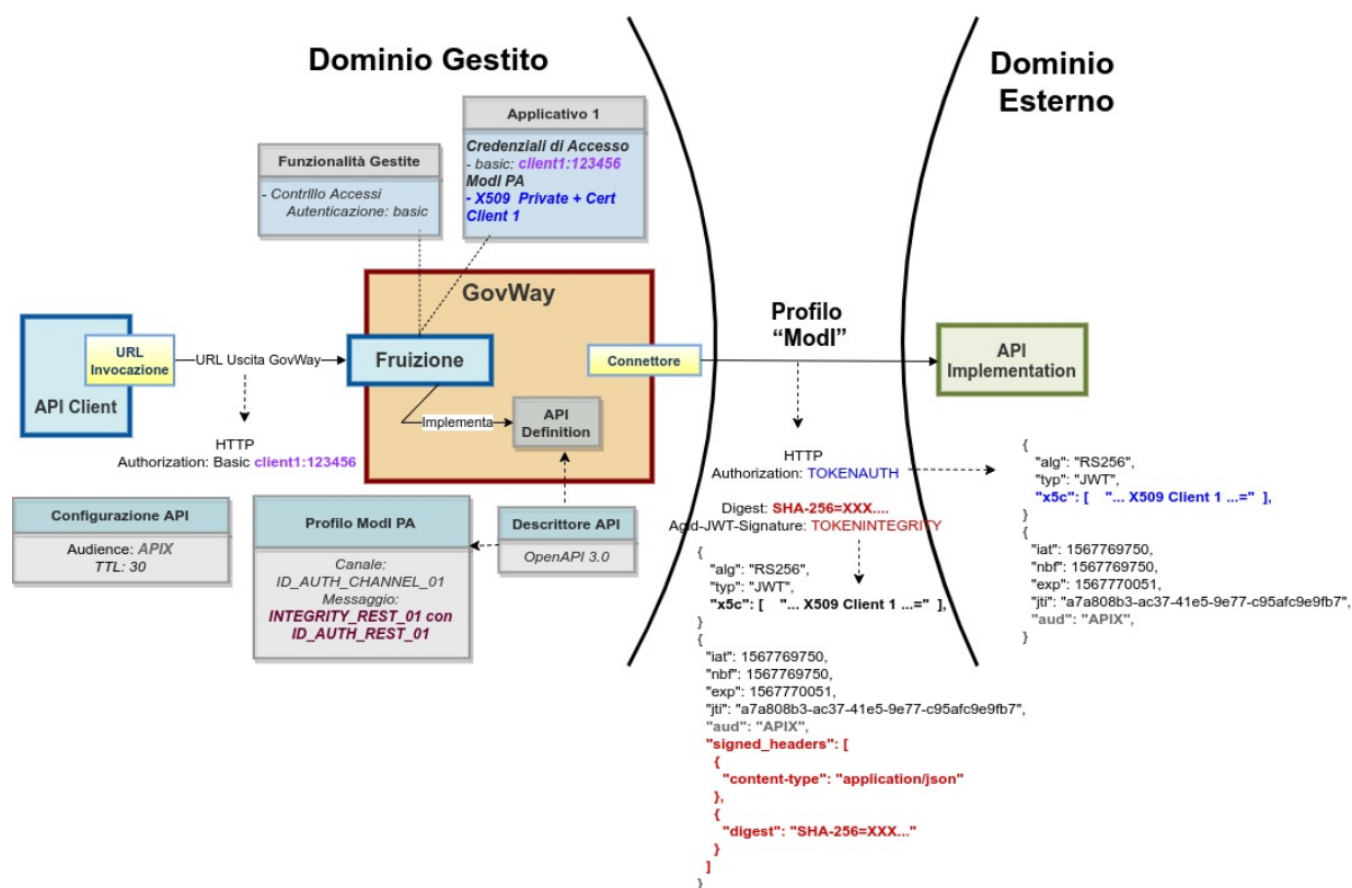
Fig. 3.82: Fruizione con Profilo di Interoperabilità "ModI", pattern "INTEGRITY_REST_01": trust tra fruitore ed erogatore tramite certificati x509
