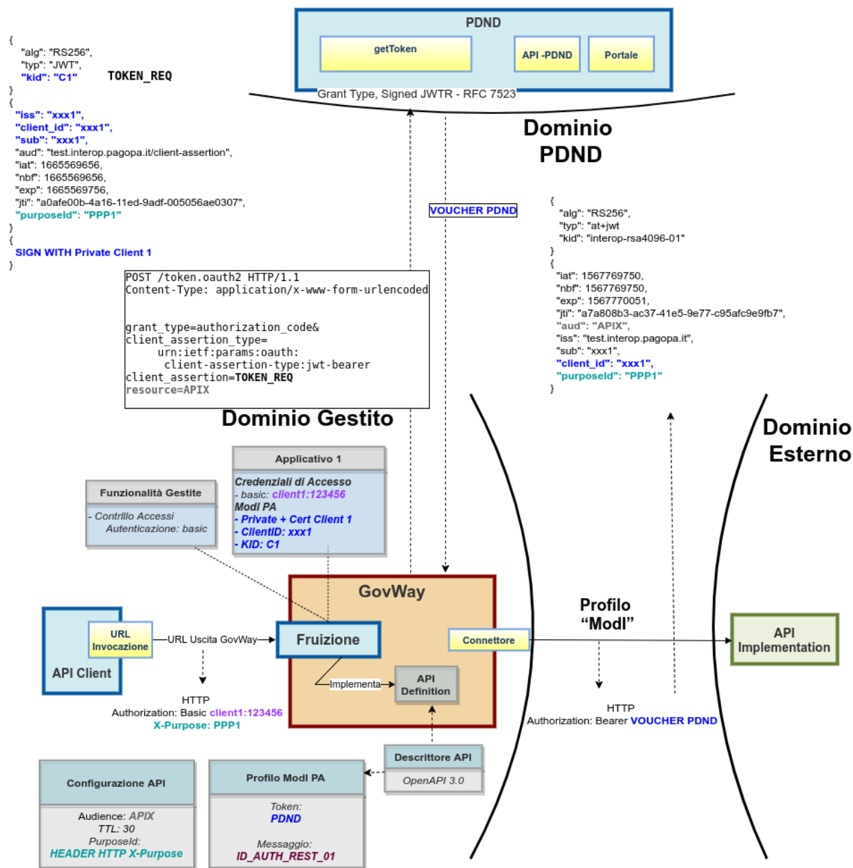
Fig. 3.16: Fruizione con Profilo di Interoperabilità "ModI", pattern "ID_AUTH_REST_01": trust tramite PDND
