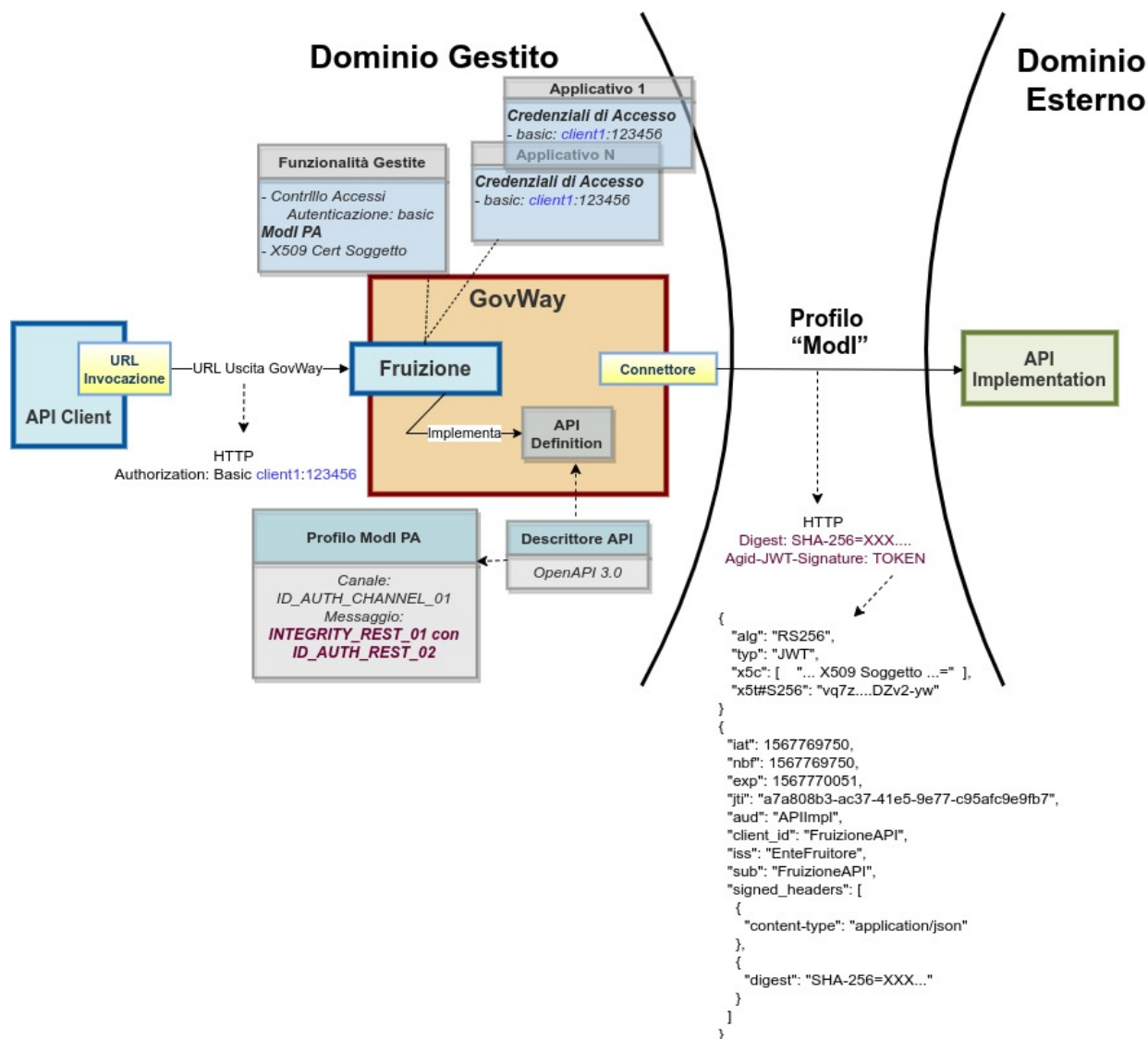
Fig. 3.123: Fruizione con Profilo di Interoperabilità "ModI"; keystore definito nella fruizione
