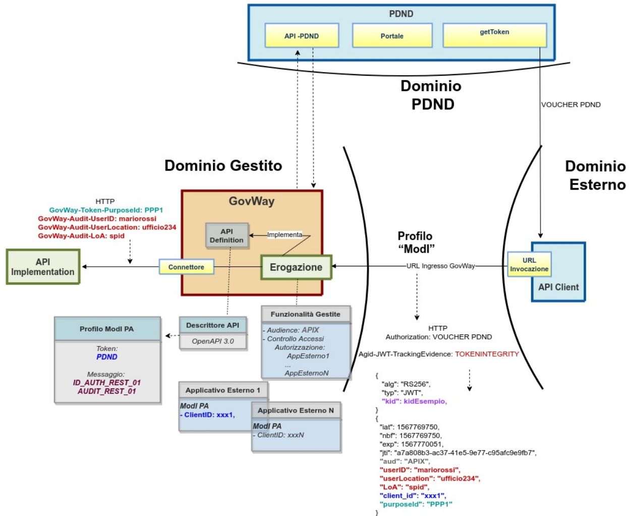
Fig. 3.97: Erogazione con Profilo di Interoperabilità “ModI”, pattern “AUDIT_REST_01”: trust tramite PDND
