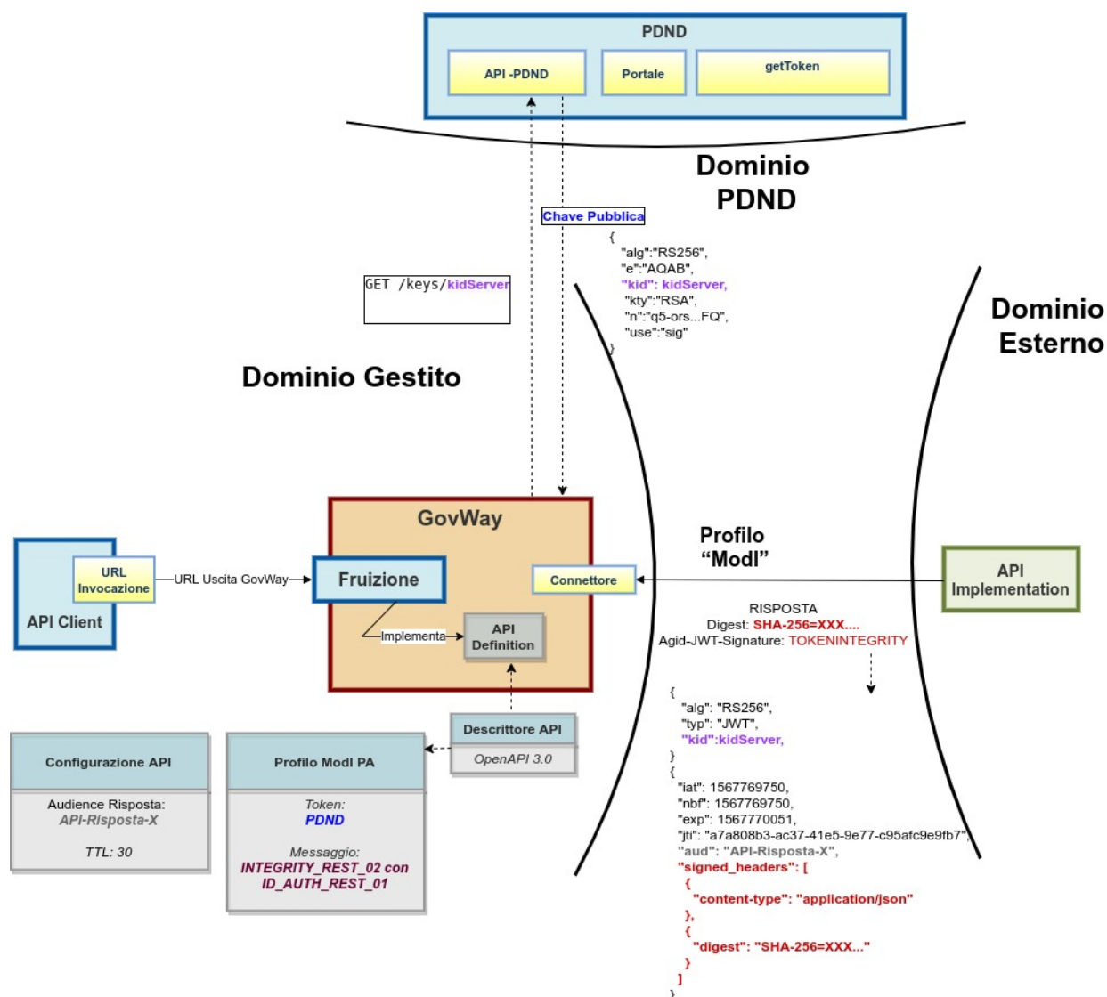
Fig. 3.74: Fruizione con Profilo di Interoperabilità “ModI”, pattern “INTEGRITY_REST_02”: trust tramite PDND e utilizzo delle API PDND per ottenere la chiave pubblica per validare la risposta
