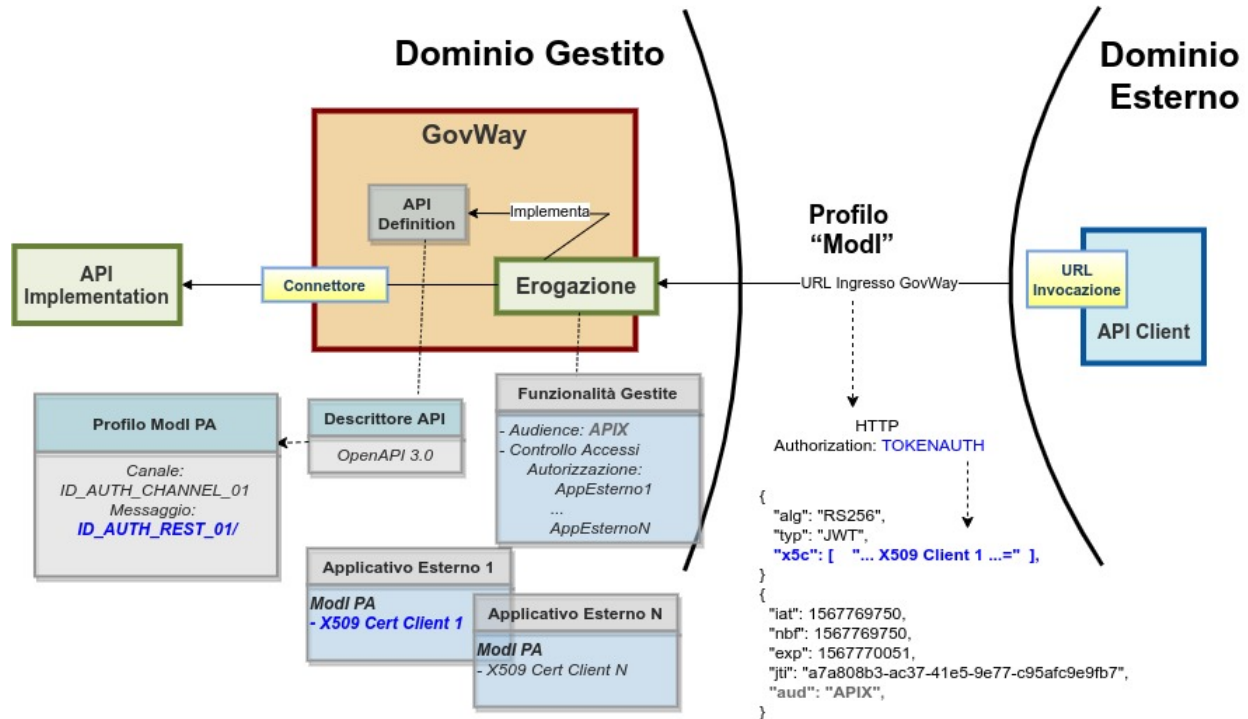
Fig. 3.54: Erogazione con Profilo di Interoperabilità “ModI”, pattern “ID_AUTH_REST_01”: trust tra fruitore ed erogatore tramite certificati x509
