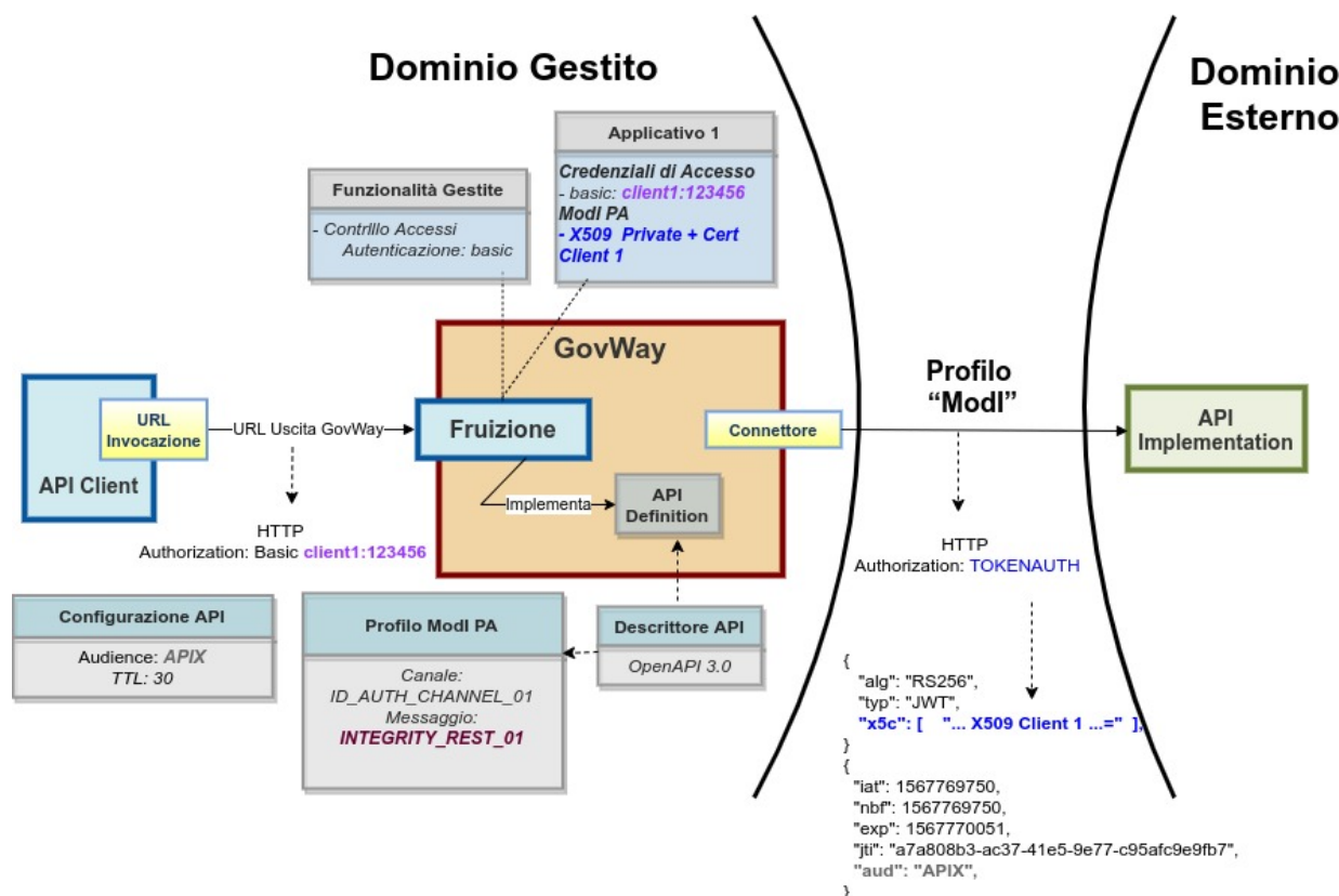
Fig. 3.50: Fruizione con Profilo di Interoperabilità “ModI”, pattern “ID_AUTH_REST_01”: trust tra fruitore ed erogatore tramite certificati x509
