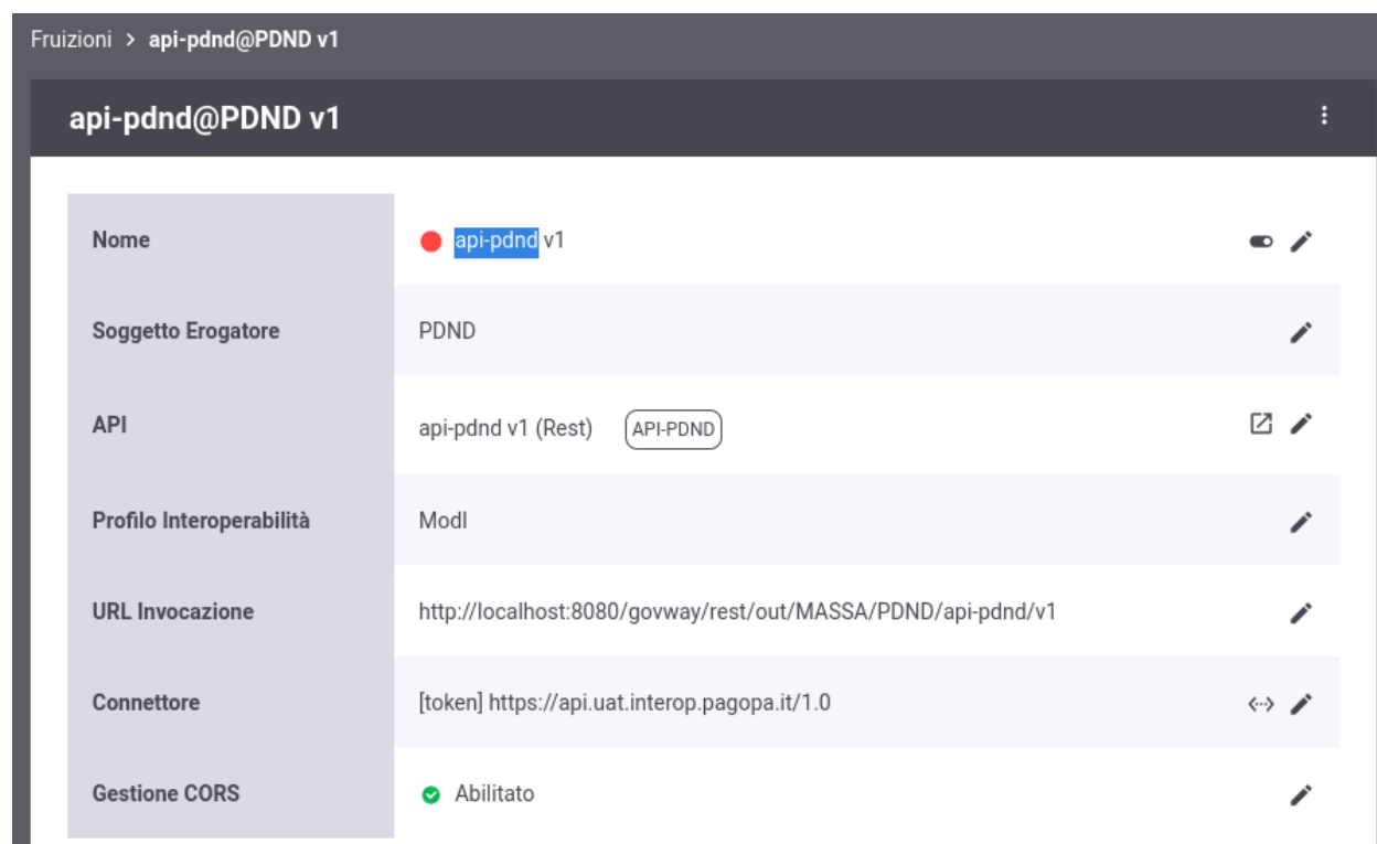
Fig. 3.12: Fruizione delle API PDND
