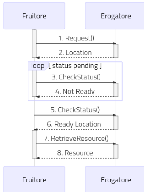
Fig. 3.145: Flusso previsto in un Pattern di Interazione PULL per API REST
