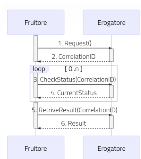
Fig. 3.139: Flusso previsto in un Pattern di Interazione PULL per API SOAP
