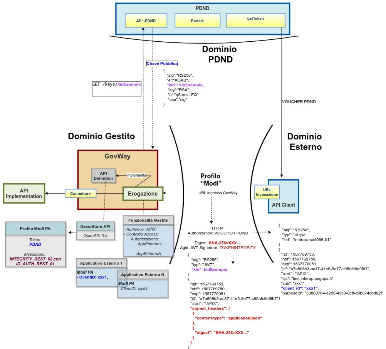
Fig. 3.75: Erogazione con Profilo di Interoperabilità "ModI", pattern "INTEGRITY_REST_02": trust tramite PDND
