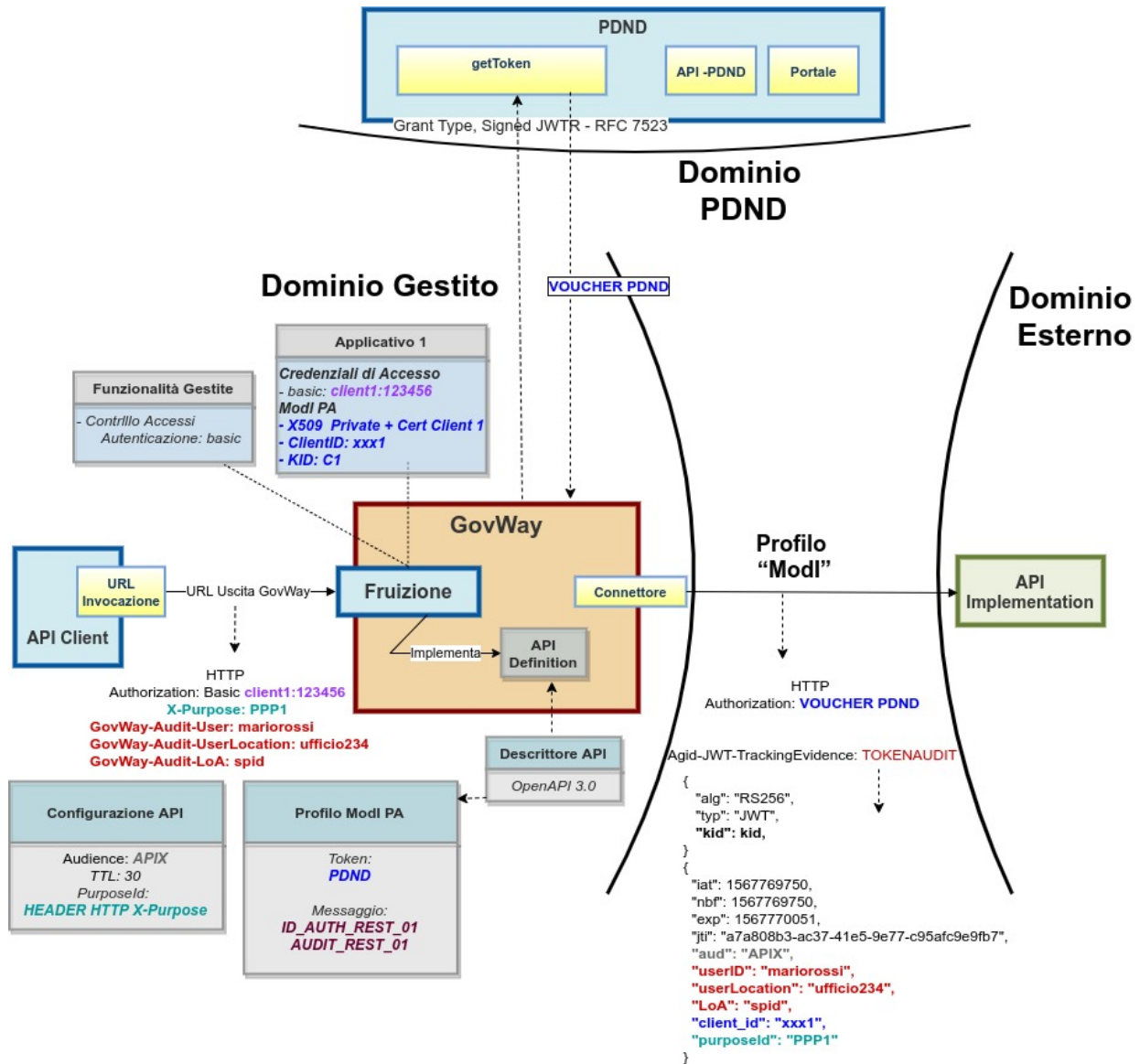
Fig. 3.94: Fruizione con Profilo di Interoperabilità “ModI”, pattern “AUDIT_REST_01”: trust tramite PDND
