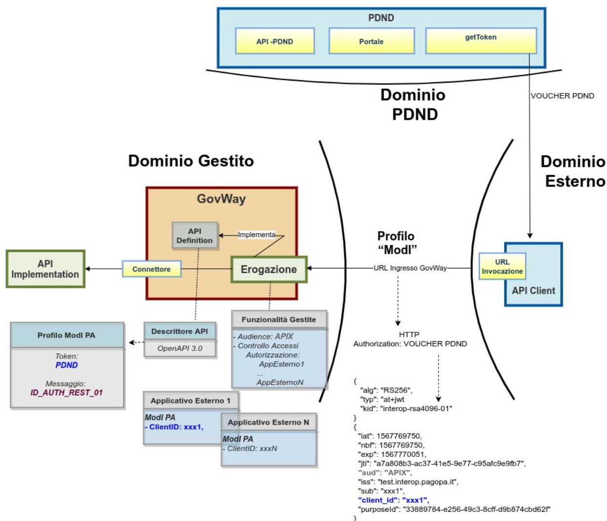
Fig. 3.39: Erogazione con Profilo di Interoperabilità “ModI”, pattern “ID_AUTH_REST_01”: trust tramite PDND
