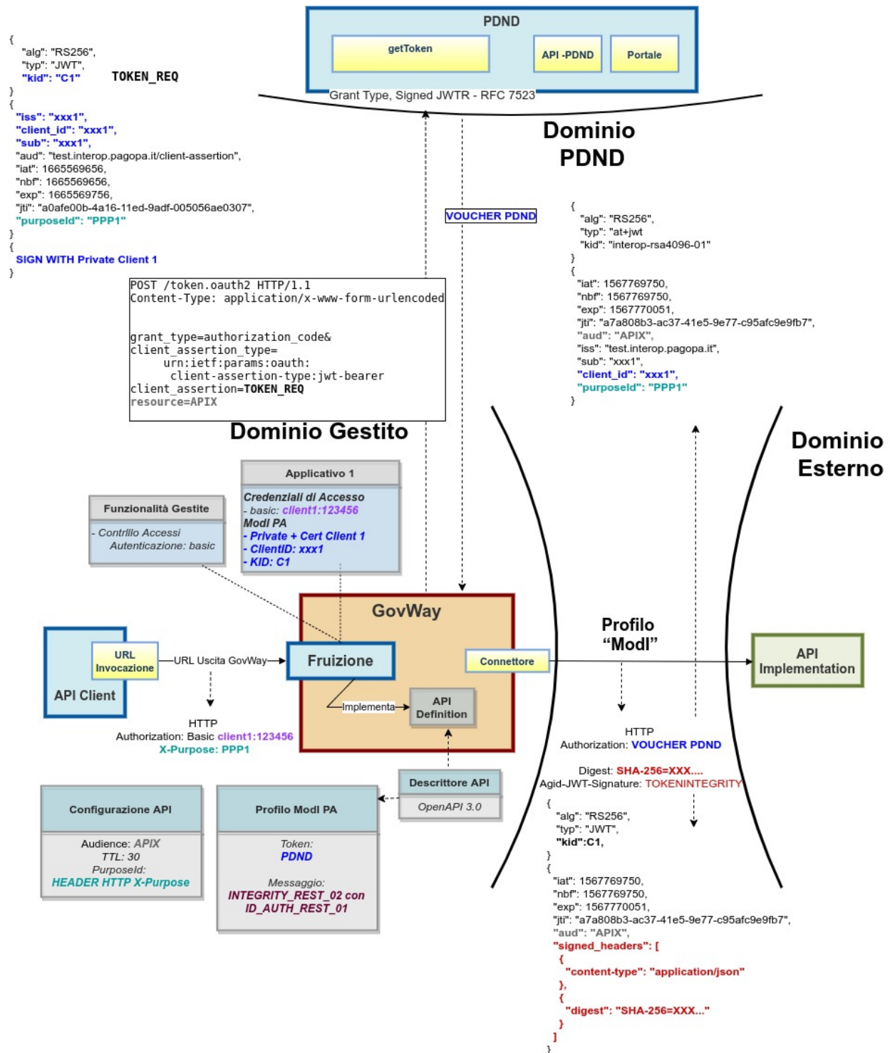
Fig. 3.69: Fruizione con Profilo di Interoperabilità "ModI", pattern "INTEGRITY_REST_02": trust tramite PDND
