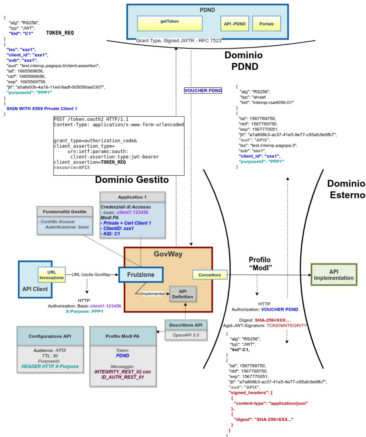
Figure3.7: Fruizione con Profilo di Interoperabilità “ModI”: trust tramite PDND
