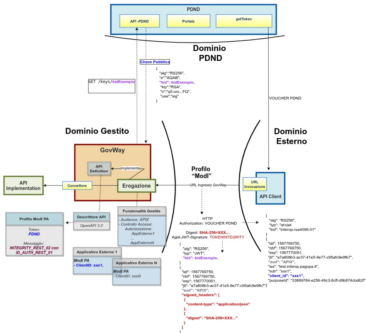
Figure3.77: Erogazione con Profilo di Interoperabilità "ModI", pattern "INTEGRITY_REST_02": trust tramite PDND
